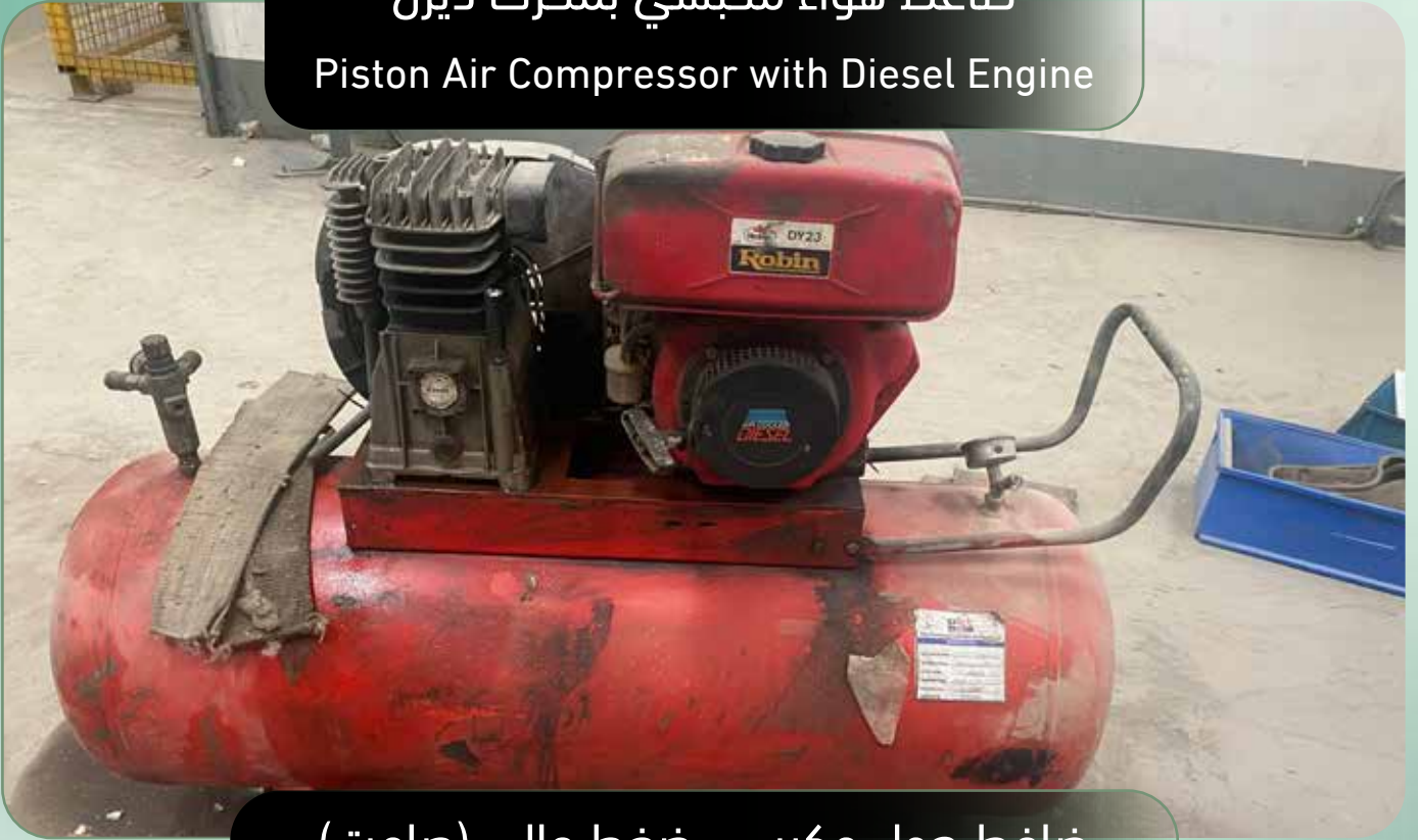
ضاغط هواء مكبسي ضغط عالي (صامت) High-Pressure Silent Piston Air Compressor
