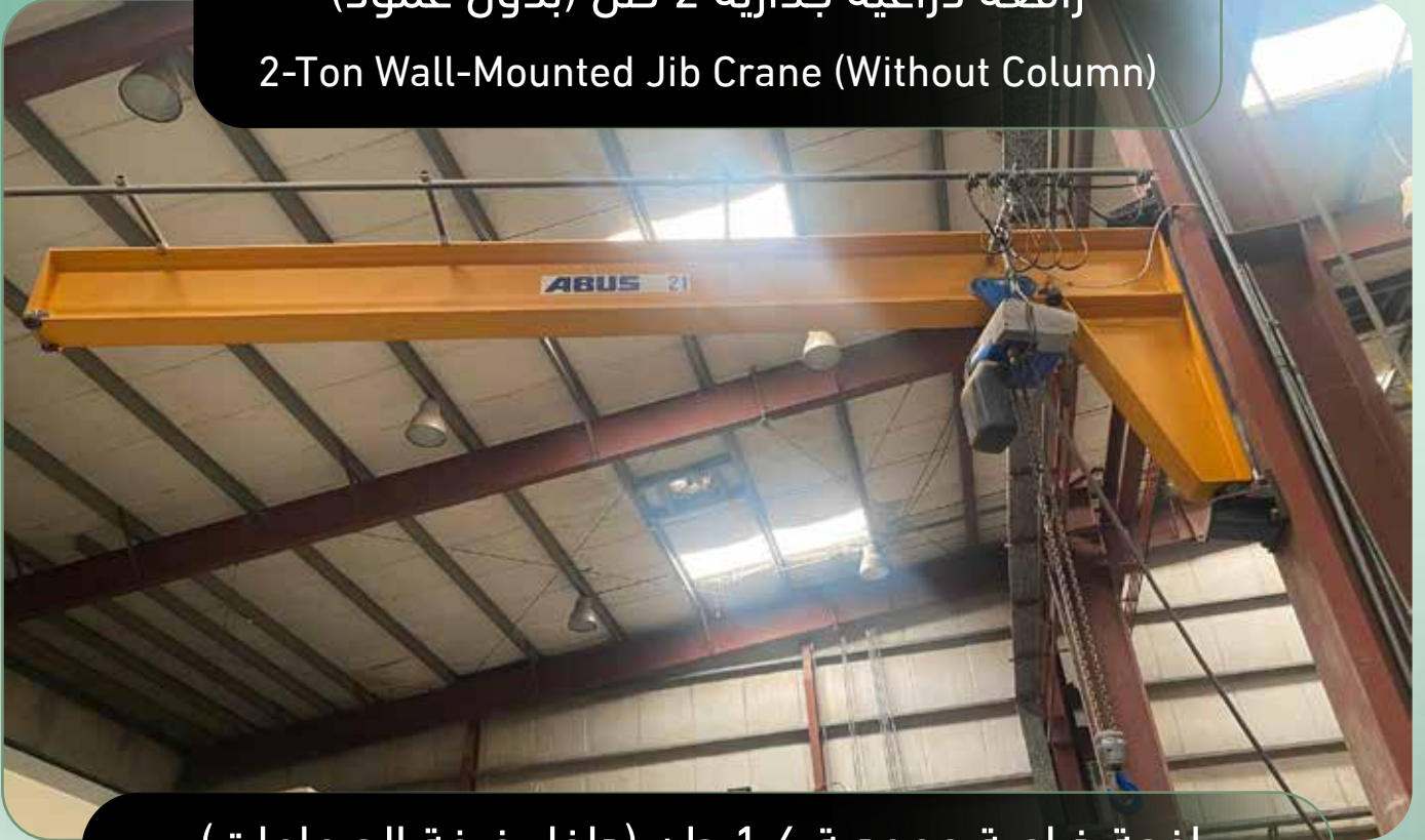
رافعة ذراعية عمودية 1.6 طن (داخل غرفة الصمامات) 1.6-Ton Column-Mounted Jib Crane (Inside the Valve Room)
